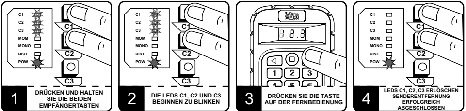
Abb. 4 Entfernen des Senders.
