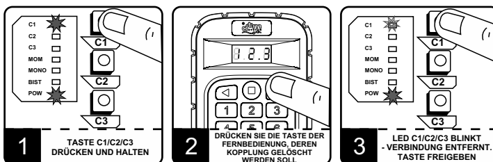
Abb. 3 Entfernen der Knopfverbindung
